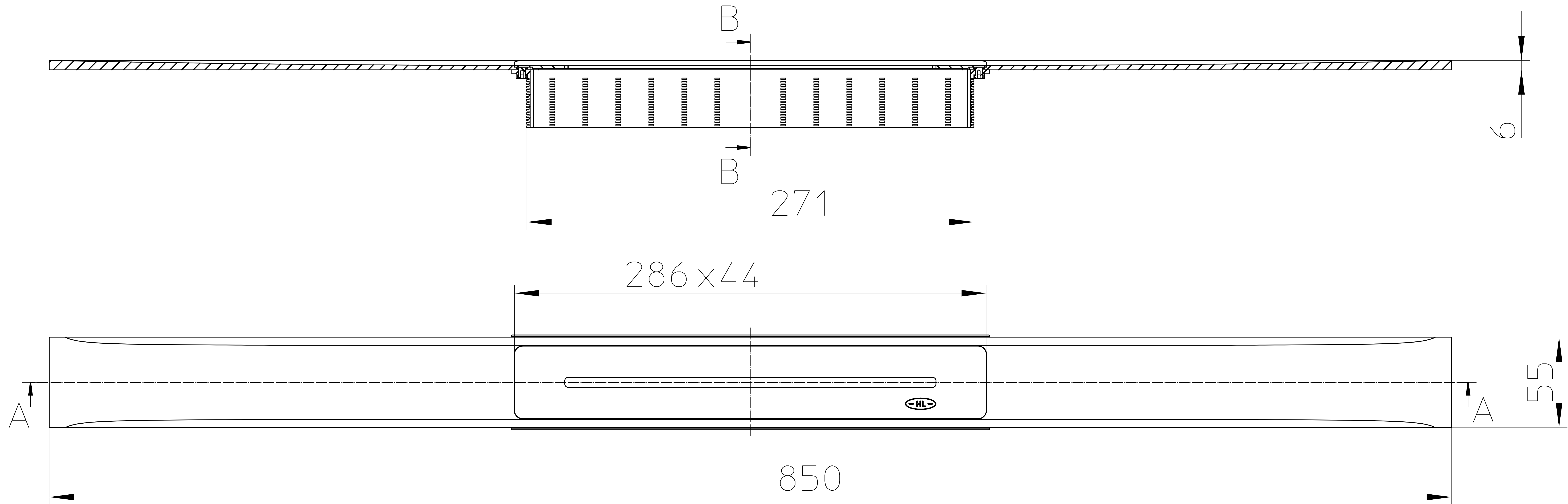
Schnitt A-A
